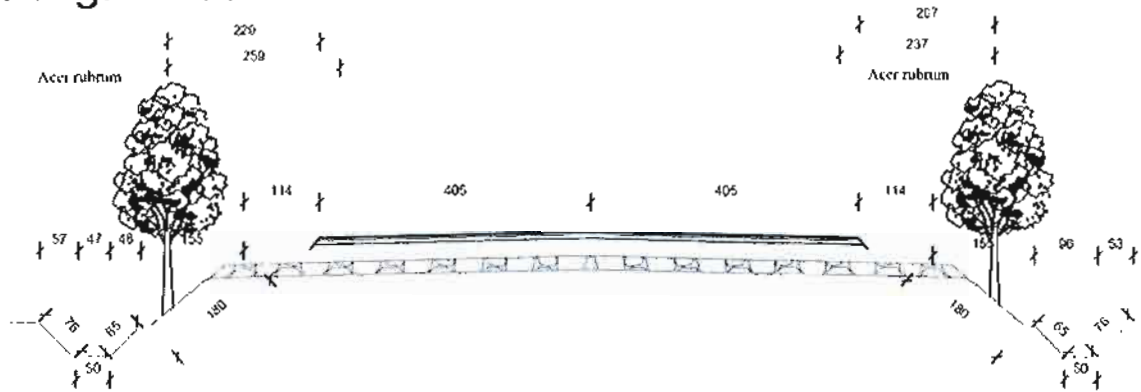
Skema 3.1.5 Profili terthor i propozuar ku paraqitet i ruga dhe gjelbërimi në të 2 krahet e saj
