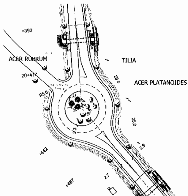
Skema 3.1. Situata e propozuar për rrethi rotullimit e gjelbëruar në 3 plan
